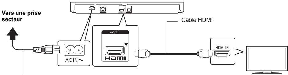
Cordon d'alimentation CA (fourni)
